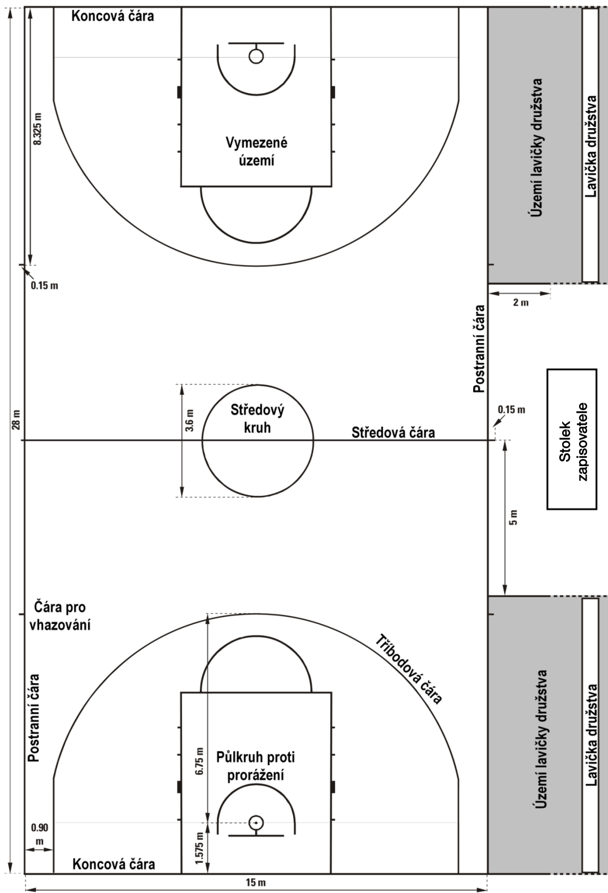
Obrázek 1 Rozměry hřiště
